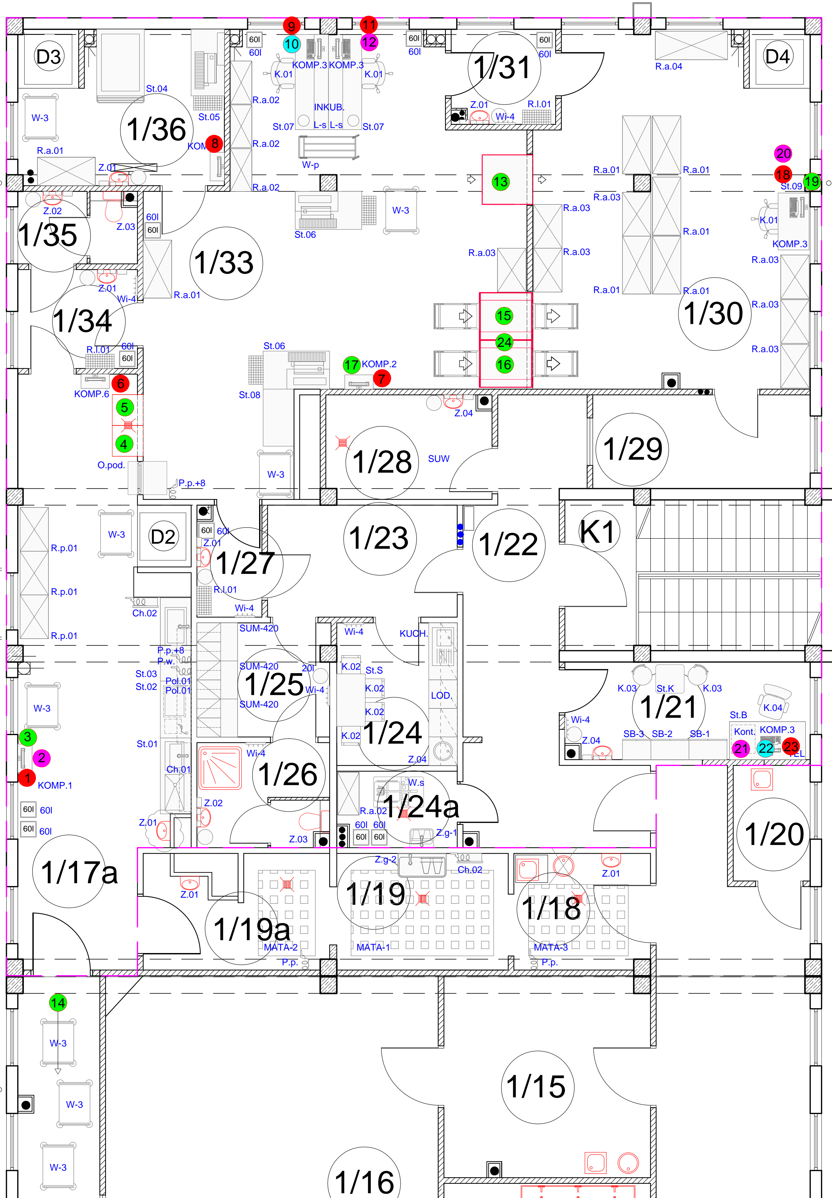
Szpital w Krotoszynie koncepcja technologii CS-001 skala 1:50 format A2
