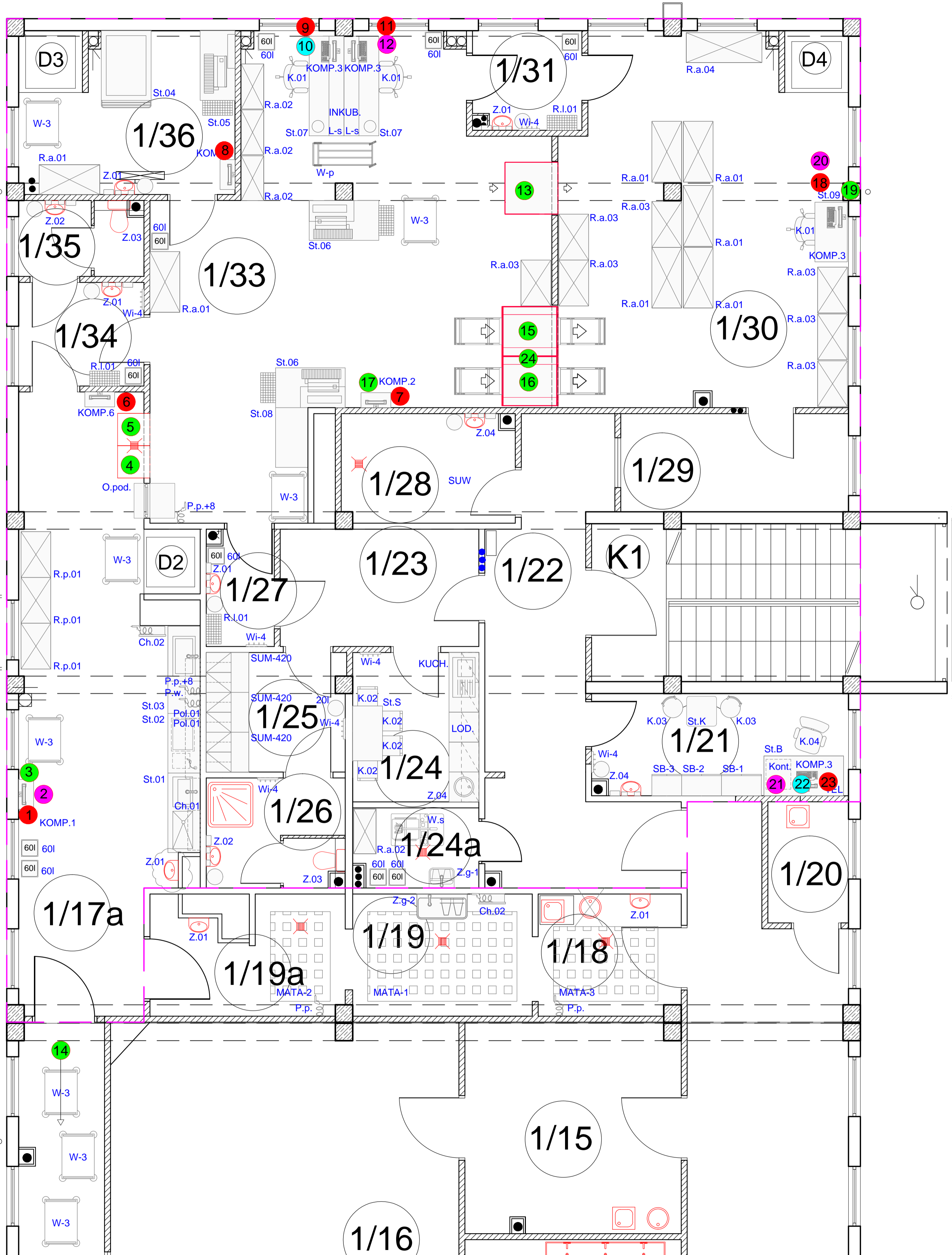
Szpital w Krotoszynie konceptja technologii CS-001 skala 1:50 format A2
